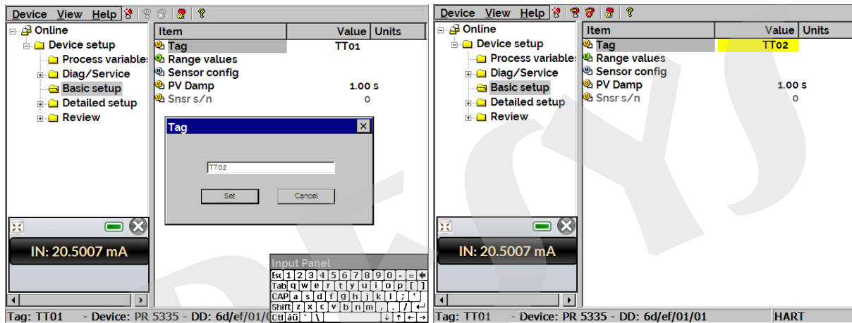
Fig. 20 - Example 2: Setting up a HART ® instrument parameter
