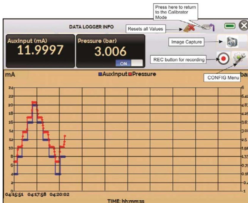
Fig. 77 – Data Logger.
