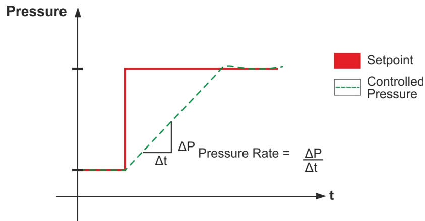
Fig. 20 – Linear control mode.
